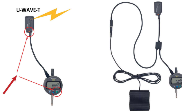
Cavo senza connettore per interruttore a pedale
